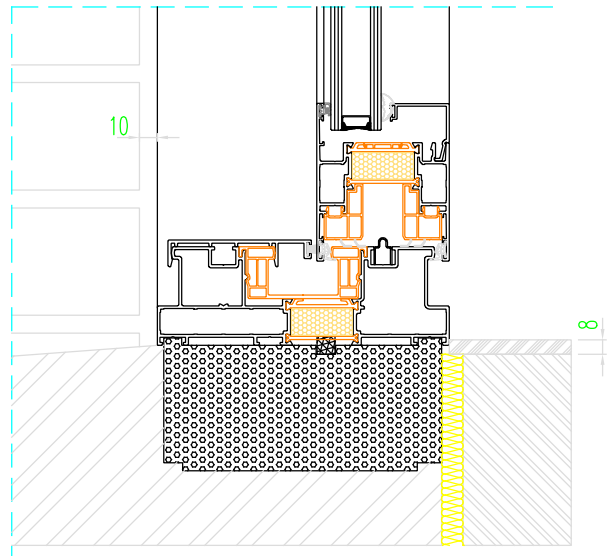
Dorpelaansluiting met P-163-92xx
