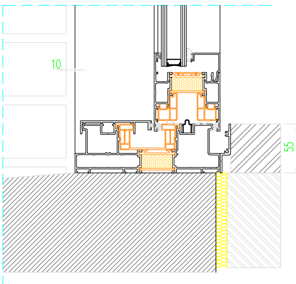
Dorpelaansluiting met P-163-5010
