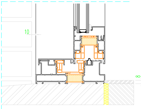
Dorpelaansluiting met P-163-92xx
