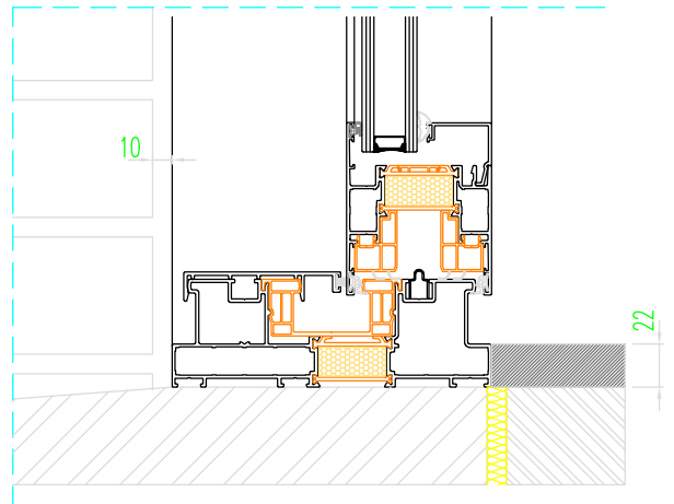
Dorpelaansluiting met P-163-92xx
